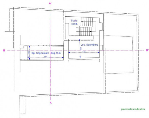
Pianta Piano Sottotetto
